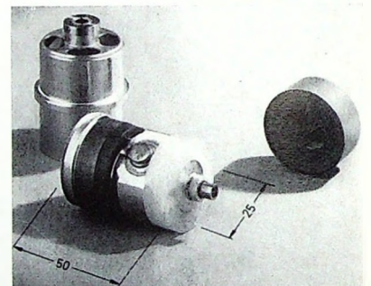
Bild 5. Wendekreisel, wie sie bei allen Raumflugaufgaben in den Raumflugkörpern verwendet werden (Aufnahme Teldix)
