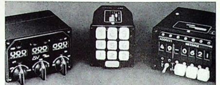
Bild 3. Numerische Anzeige, Eingabegerät und Geschwindigkeitsanzeige für das Rendezvousmanöver des Führungsrechners, wie er bereits im Gemini-Programm benutzt wurde (Aufnahme IBM)
