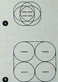
Bild 17. Überlagerung der Feldverteilung in der virtuellen Apertur bei vier Einzelanordnungen (Yagi-antennen): a) bei relativ geringem gegenseitigen Abstand, b) bei optimalem gegenseitigen Abstand
