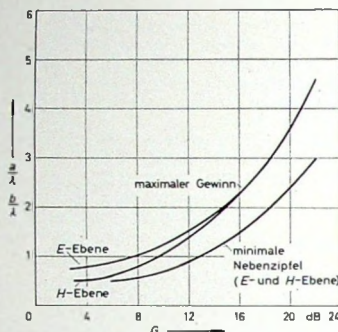
Bild 12. Erforderlicher gegenseitiger Abstand von Yagiantennen als Grundantennen in einer Mehrfach-Antennenanordnung als Funktion des Gewinns der Grundantenne für maximalen Gewinn bei Anordnung in der E- oder H-Ebene und für minimale Nebenzipfel in der E- und H-Ebene (Näherungsdimensionierung)
