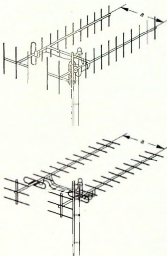
Bild 8. Praktischer Aufbau einer Antennenzeile aus zwei Yagi-Antennen mit gegenseitigem Abstand a für horizontale und vertikale Polarisation
