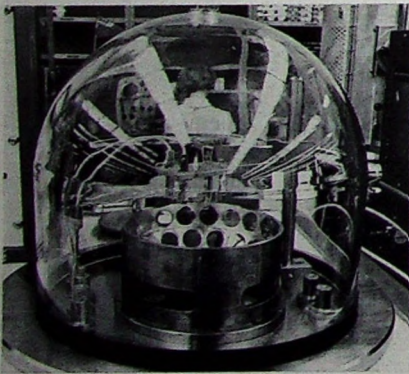
Bild 4. Aufdampfen der elektrischen Leitungswege
