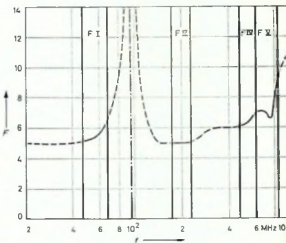
Bild 3. Rauschzahl F des Verteilungsverstärkers
