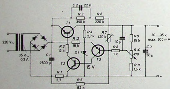
Bild 1. Schaltung des geregelten Speisegerätes; eine Brummkompensation im Rückkopplungszweig ergibt eine Restwelligkeit von weniger als 100 \mu\text{V}
