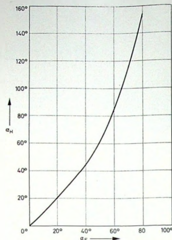
Bild 13. Näherungsweise Zusammenhang zwischen den Öffnungswinkeln der Hauptkeule bei Yagiantennen in der E- und H-Ebene
