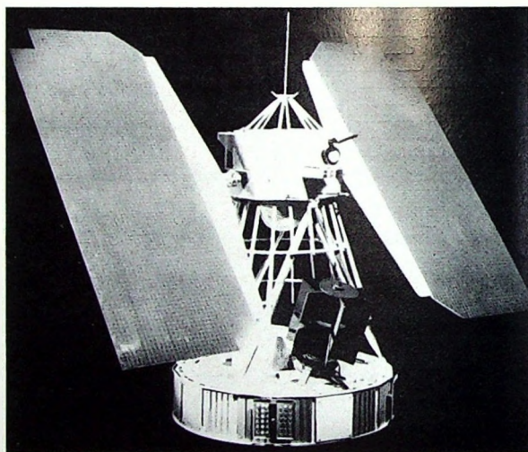
Bild 4. Modell des Nimbus 3. Deutlich erkennbar sind die Sonnenpaddel, der Atomreaktor, der kugelförmige Stickstoffbehälter für die Lagestabilisierung und (oben) eine stablförmige Antenne, darunter Stickstoffdüsen
