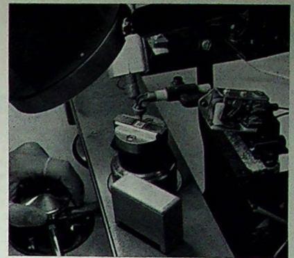
Bild 12. Kontaktierung der einzelnen Schaltungen
