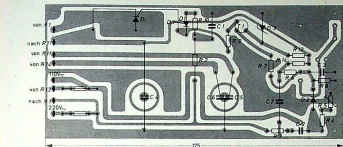
Bild 6. Gedruckte Platte zum phasenanschnittgesteuerten Thyristor-Netzteil nach Bild 4
