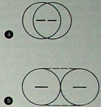
Bild 16. Überlagerung der Feldverteilung in der virtuellen Apertur von zum Beispiel Yagi-antennen und resultierende Feldverteilung: a) bei relativ geringem gegenseitigen Abstand, b) bei optimalem gegenseitigen Abstand
