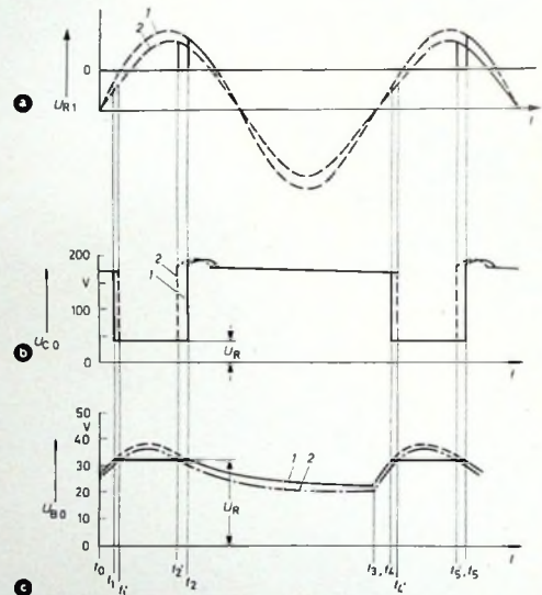
Bild 5. Spannungsverläufe beim phasenschnittgesteuerten Thyristor-Netzteil nach Bild 4: a) Spannung U_{R1} am Vorwiderstand R1 , b) Kollektorspannung U_{C0} des Transistors T1 , c) Basisspannung U_{B0} des Transistors T1
