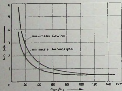
Bild 11. Erforderlicher gegenseitiger Abstand von beliebigen Grundantennen in einer Mehrfach-Antennenanordnung als Funktion des Öffnungswinkels der Hauptkeule der Einzelantenne für maximalen Gewinn oder minimale Nebenzipfel (Näherungsdimensionierung der Mehrfachantennenanordnung)
