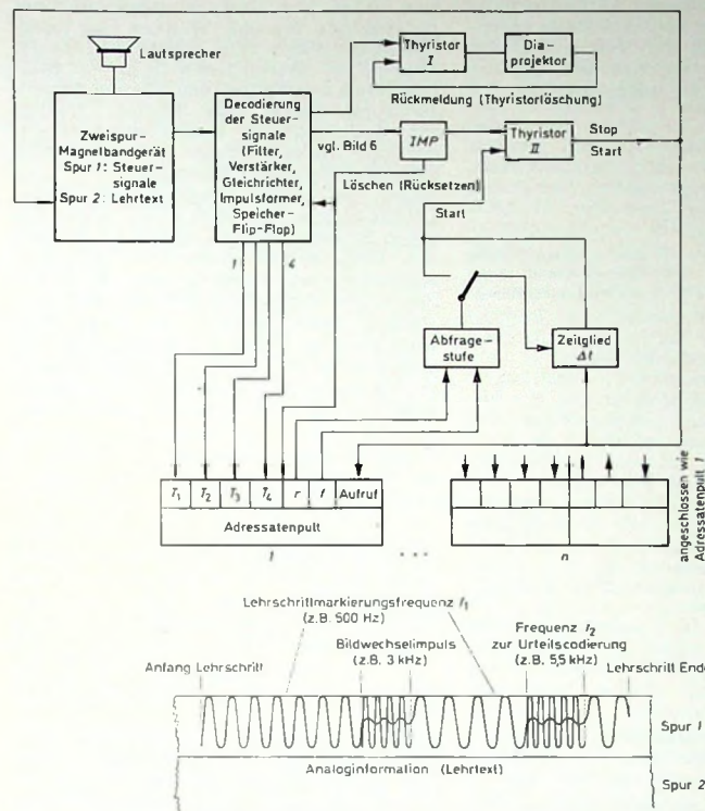
Bild 3. Beispiel eines einfachen Lehrautomaten ohne Rechner (Prinzip)
