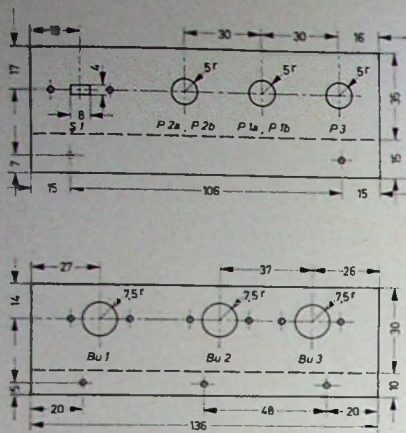
Bild 6. Maßskizzen (Frontplatten und Rückseite)
