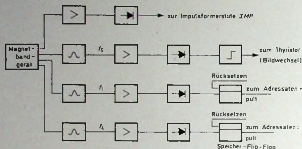
Bild 6. Vereinfachtes Blockschaltbild einer Decodiereinrichtung
